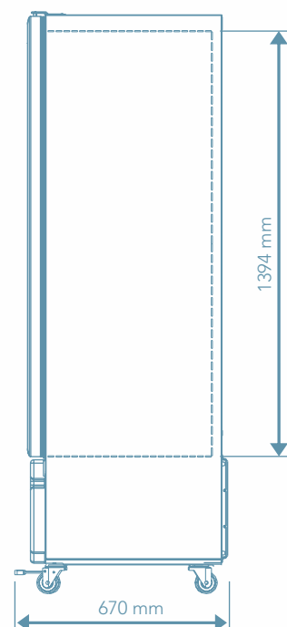
VISTA LATERAL
